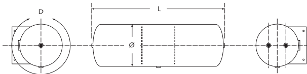
Tekening (C)
